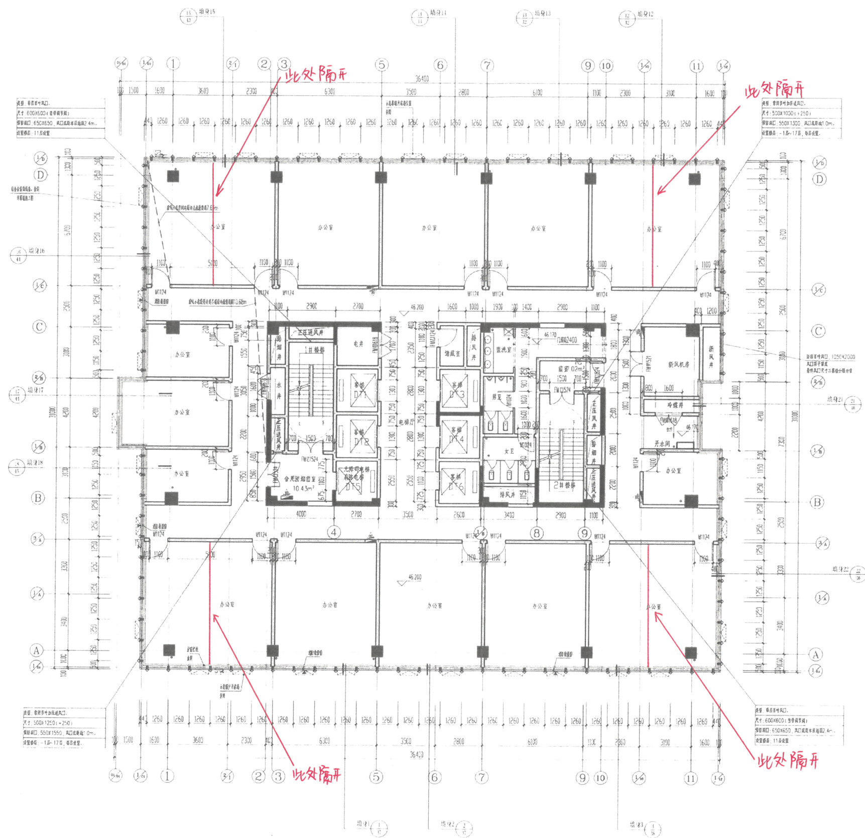
十一层平面图 1:100
