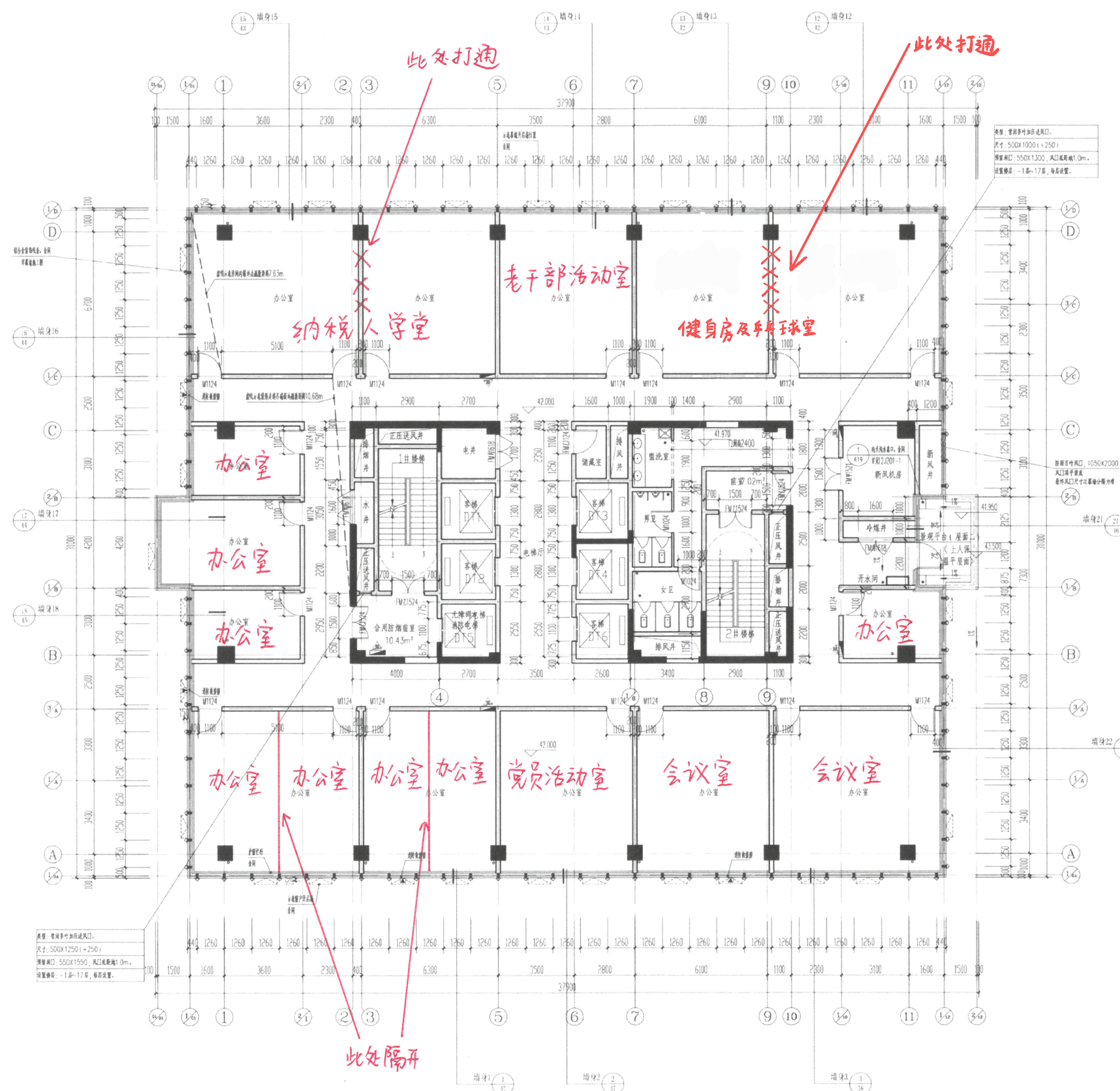
十层平面图 1:100
